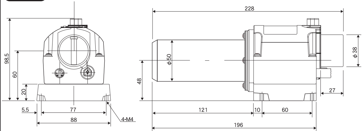
寸法図
