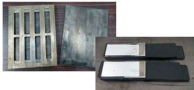
JIS K 6256-2 試験片および金型
